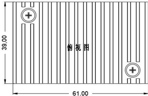
标准型+散热器 61.0*39.0*27.7mm
