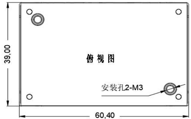
标准型 60.4*39.0*12.7mm
