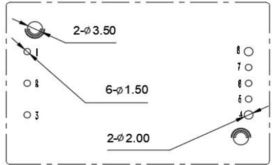
推荐PCB开槽尺寸
